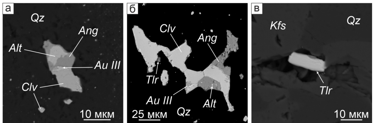
Рис. 4.17. Англезит, теллурит и ассоциирующие с ними минералы: а – англезит, замещающий алтаит; б – англезит, замещающий алтаит, а также теллурит, замещающий калаверит совместно с «горчичным» самородным золотом III; в – столбчатый кристалл теллурита в полости в жильном калиевополевошпат-кварцевом агрегате. Изображения в обратно-рассеянных электронах. Qz – кварц, Ang – англезит, Alt – алтаит, Au III – самородное золото третьей разновидности («горчичное» золото), Clv – калаверит, Tlr – теллурит, Kfs – калиевый полевой шпат.
