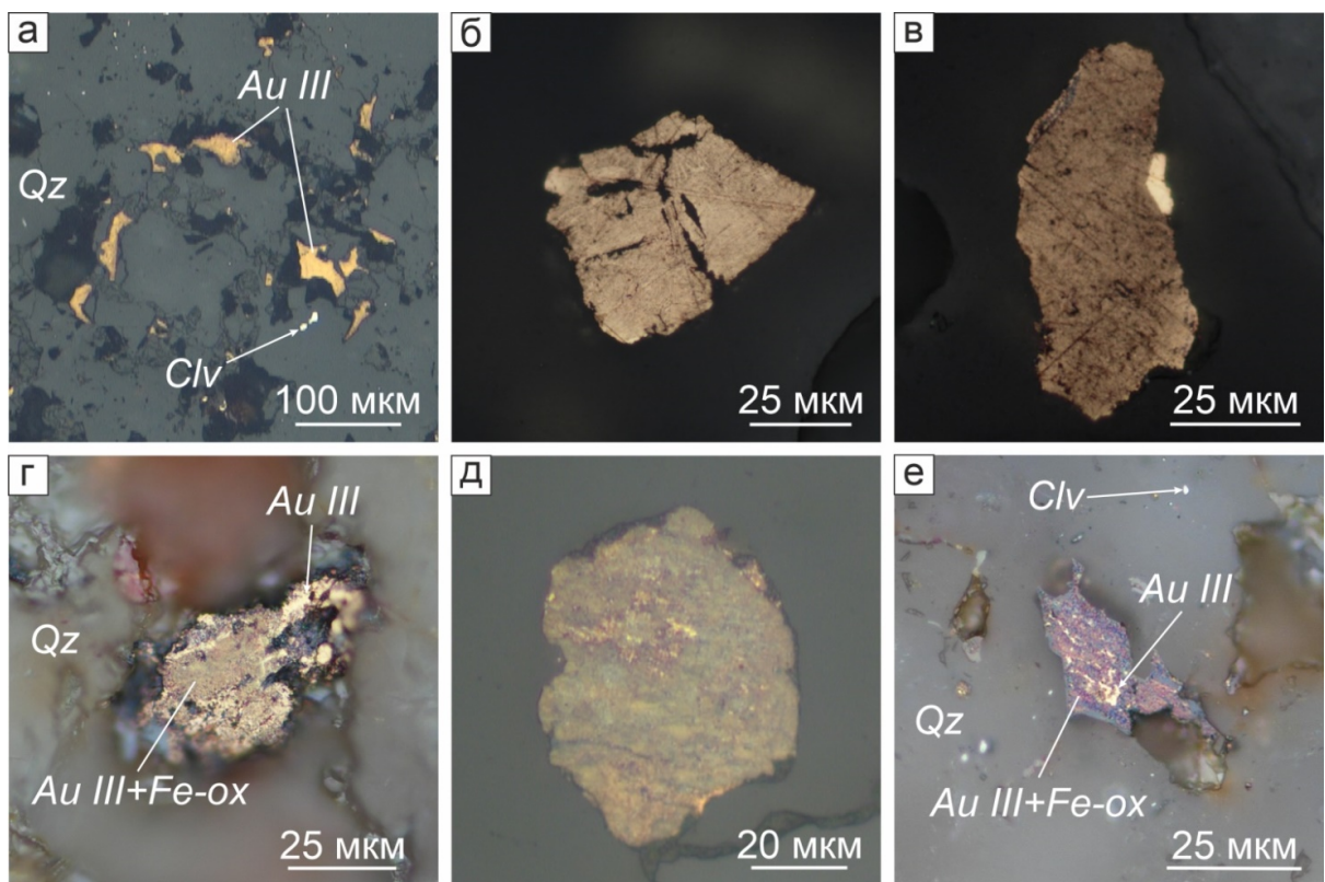
Рис. 4.12. Самородное золото III («горчичное» золото), особенности его внутреннего строения и взаимоотношения с другими минералами: а – скопление угловатых зерен «горчичного» золота в полостях калиевополевошпат-кварцевой матрицы; б – трещиноватое зерно «горчичного» золота; в – пористое неоднородное зерно «горчичного» золота с участком золота, свободного от примесей (светлое); г–е – неоднородные зерна «горчичного» золота, в которых темные участки насыщены примесями, а светлые – обеднены примесями. Изображения в отраженном свете. Au III – самородное золото третьей разновидности («горчичное» золото), Qz – кварц, Clv – калаверит, Fe-ox – гидроксиды железа.
