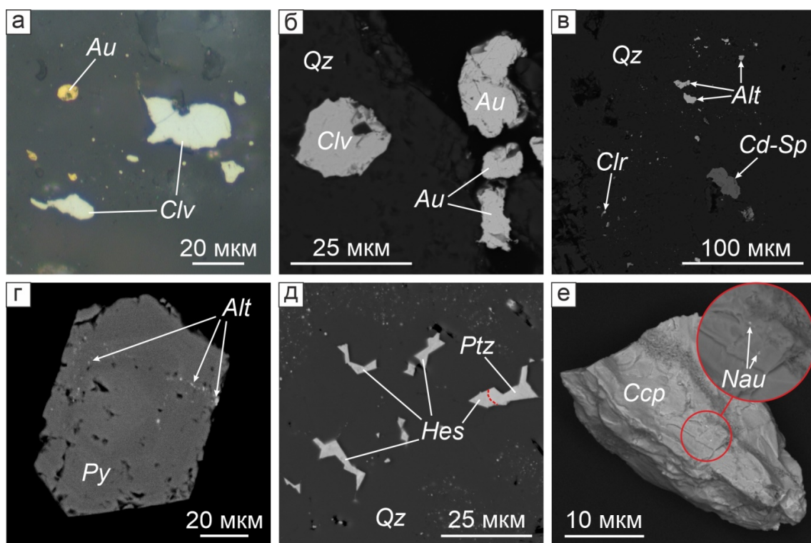
Рис. 4.6. Теллуриды, селениды, их морфология, внутреннее строение зерен и взаимоотношения с другими минералами: а, б – ассоциация калаверита и самородного золота; в – ассоциация алтаита, колорадоита и кадмийсодержащего сфалерита в кварце; г – вкрапленность алтаита в кристалле пирита; д – угловатые ксеноморфные зерна гессита и петцита, а также тонкая «эмульсионная» вкрапленность этих же и других теллуридов (белые точки) в кварце; е – вкрапленность науманнита в халькопирите. Фото в отраженном свете (а), изображения в обратно-рассеянных электронах (б–д) и во вторичных электронах (е). Au – самородное золото, Clv – калаверит, Qz – кварц, Alt – алтаит, Clr – колорадоит, Cd-Sp – кадмийсодержащий сфалерит, Ptz – петцит, Hes – гессит, Ccp – халькопирит, Nau – науманнит.
