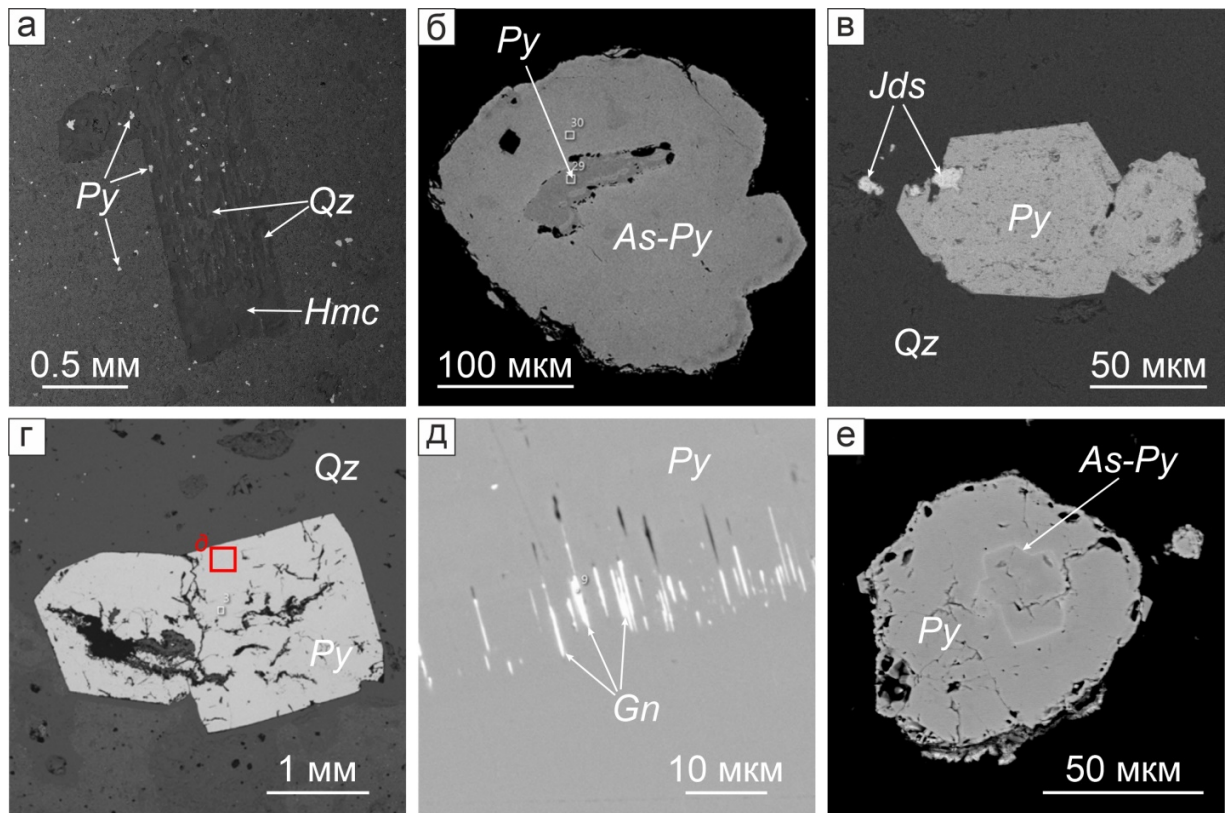
Рис. 4.19. Особенности морфологии и внутреннего строения зерен пирита: а – рассеянная вкрапленность пирита в аргиллите; б – кристалл мышьяксодержащего пирита округлой формы на затравке резорбированного пирита; в – включение йордизита в пирите; г, д – крупное зерно пирита с включениями галенита по зоне роста; е – пирит с зоной роста, насыщенной мышьяком. Изображения в обратно-рассеянных электронах. Py – пирит, Qz – кварц, Hmc – минералы группы гидрослюд, As-Py – мышьяксодержавший пирит, Jds – йордизит, Gn – галенит.
