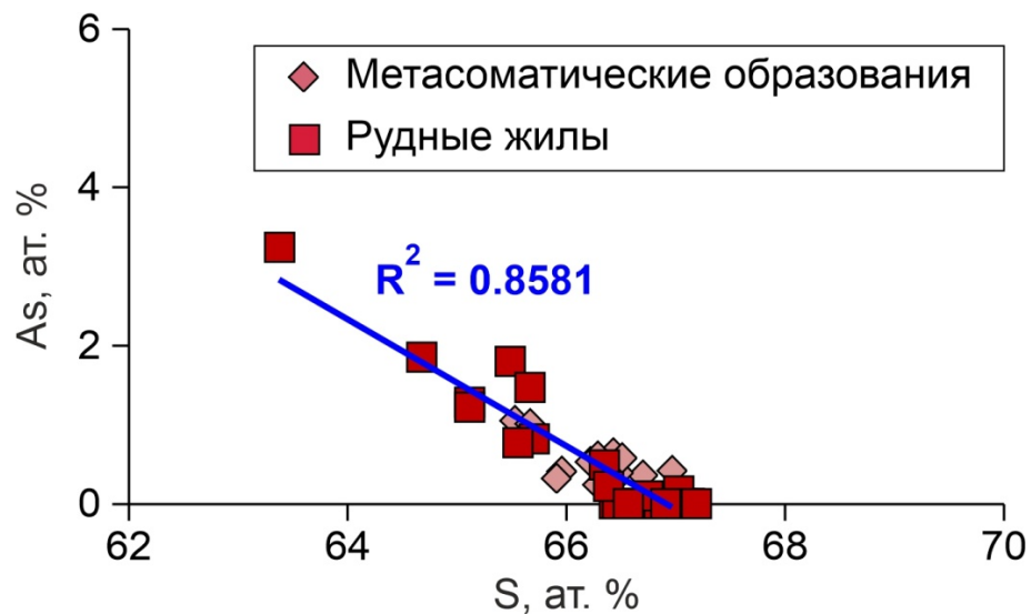
Рис. 4.20. Обратная корреляционная зависимость между содержанием S и As в пирите, участок Северный. R^2 – коэффициент детерминации.
