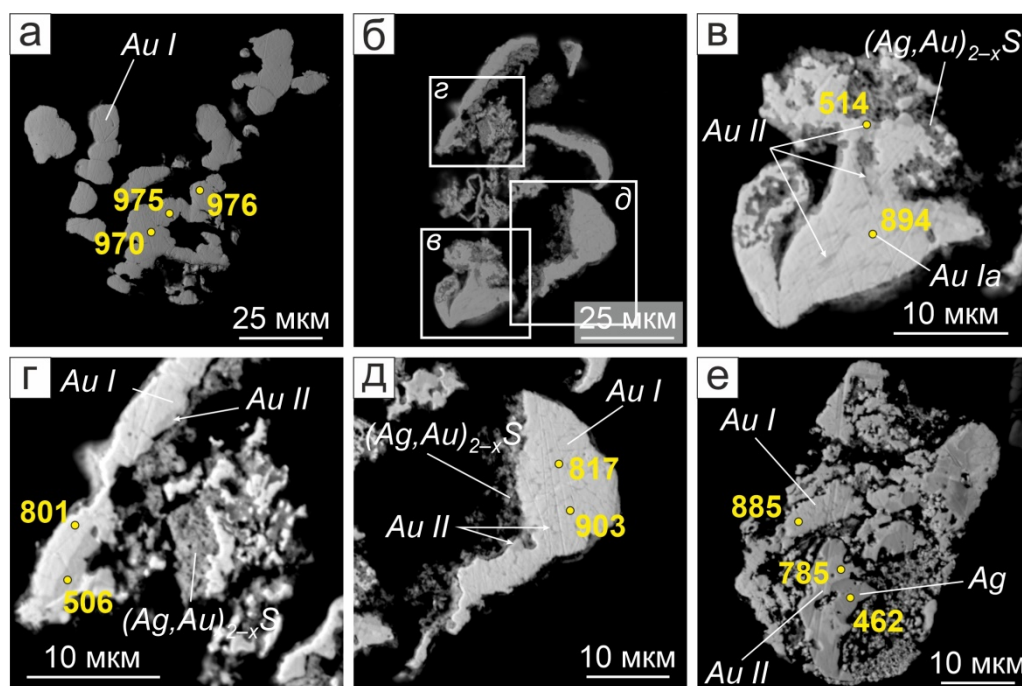
Рис. 4.10. Внутреннее строение дендритовидных агрегатов самородного золота I и II: а – дендритовидное зерно высокопробного самородного золота с однородным внутренним строением; б–д – зерно неоднородного внутреннего строения, в котором различные участки сложены самородным золотом I и II, а каймы – фазами (Ag,Au)_{2-x}S (в–д – участки детализации); е – зерно неоднородного внутреннего строения, в котором различные участки сложены самородным золотом I, II и самородным серебром. Изображения в обратно-рассеянных электронах. На изображениях а, в–е желтые круги – аналитические точки, числа – пробность золота (в ‰). Au I – самородное золото первой разновидности, Au II – самородное золото второй разновидности, Ag – самородное серебро.
