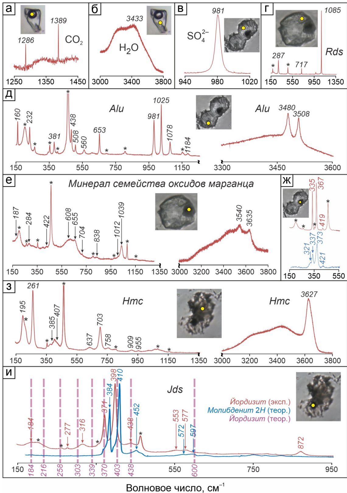
Рис. 5.3. Представительные КР-спектры флюидных включений при комнатной температуре: а – углекислый газ ( \text{CO}_2 ); б – вода ( \text{H}_2\text{O} ); в – сульфат-ион ( \text{SO}_4^{2-} ); г – родохрозит ( Rds ); д – минерал группы алунита ( Alu ); е – минерал семейства оксидов марганца; ж – аргентопирит (красный спектр – экспериментальный, синий – из базы данных RRUFF # R070173 ( http://rruff.info )); з – минерал группы гидрослюд ( Hmc ); и – йордизит ( Jds ) (красный спектр – экспериментальный, синий – из базы данных RRUFF # R050209 ( http://rruff.info ), фиолетовые полосы соответствуют положению полос йордизита по (Chukanov, Vigasina, 2020)). На фото-миниатюрах желтыми кругами обозначены аналитические точки. *Пики кварца.
