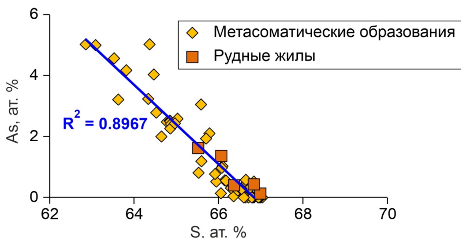
Рис. 4.3. Обратная корреляционная зависимость между содержанием S и As в пирите, участок Центральный. R^2 – коэффициент детерминации.
