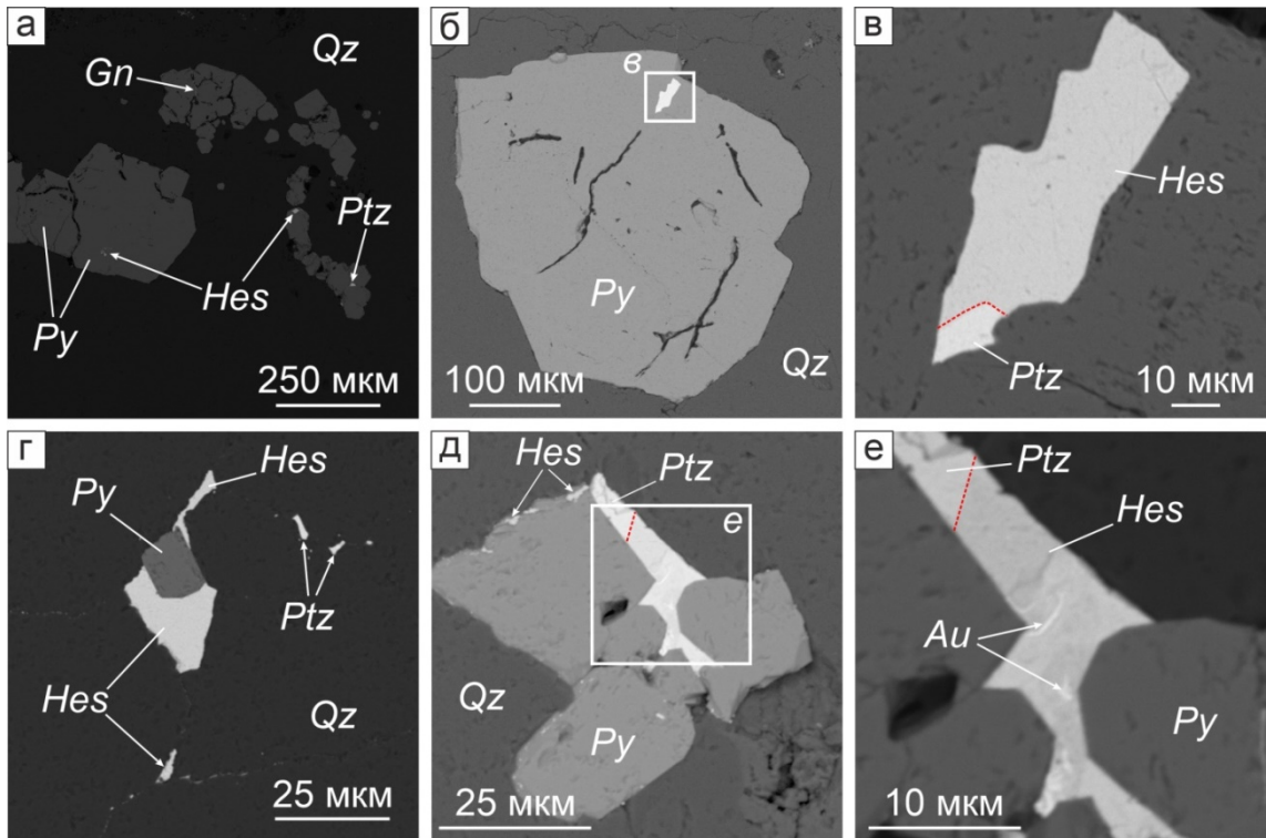
Рис. 4.23. Теллуриды, их морфология, внутреннее строение зерен и взаимоотношения с другими минералами: а – пирит с включениями петцита, гессита и галенита; б, в – включение гессита и петцита в пирите; г – пирит, обрастающий гесситом; д, е – гессит, петцит и самородное золото, в сростаниях с пиритом. Изображения в обратно-рассеянных электронах. Gn – галенит, Qz – кварц, Ptz – петцит, Hes – гессит, Py – пирит, Au – самородное золото.
