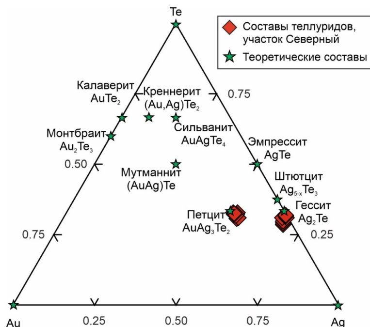
Рис. 4.24. Диаграмма составов (ат. %) минералов системы Au–Ag–Te, участок Северный, рудопроявление Эвепента.
