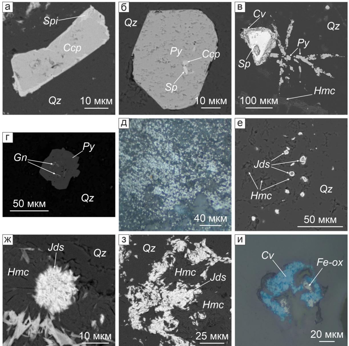
Рис. 4.21. Сульфиды, их морфология, внутреннее строение зерен и минеральные взаимоотношения: а – зерно халькопирита с каймой спонкопита (?); б – включения халькопирита и сфалерита в пирите; в – сфалерит с каймой ковеллина в ассоциации с пиритом в калиевополевошпат-кварцевом метасоматите; г – включение галенита в пирите; д – участок кварцевого прожилка, насыщенный йордизитом (коричневато-серый); е, ж – сферолитоподобные агрегаты йордизита в срастании с гидрослюдами; з – чашуйчатые кристаллы йордизита в срастании с гидрослюдами; и – агрегат ковеллина с гидроксидами железа. Фото в отраженном свете (д, и) и изображения в обратно-рассеянных электронах (а–г, е–з). Spi – спонкопит, Ccp – халькопирит, Qz – кварц, Sp – сфалерит, Cv – ковеллин, Hmc – минералы группы гидрослюдов, Gn – галенит, Jds – йордизит, Fe-ox – гидроксиды железа.
