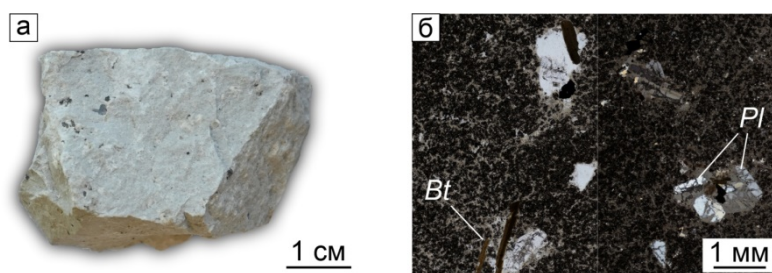
Рис. 3.1. Вмещающие риодациты: а – образец риодацита; б – микрофотография риодацита в петрографическом шлифе (слева – без анализатора, справа – под анализатором). Bt – биотит, Pl – плагиоклаз.
