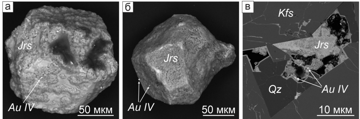
Рис. 4.14. Морфологические особенности самородного золота IV: а, б – самородное золото IV на поверхности псевдоморфоз ярозита по пириту; в – вкрапленность самородного золота IV в ярозите. Изображения во вторичных электронах (а, б) и в обратно-рассеянных электронах (в). Jrs – ярозит, Au IV – самородное золото четвертой разновидности, Kfs – калиевый полевой шпат, Qz – кварц.
