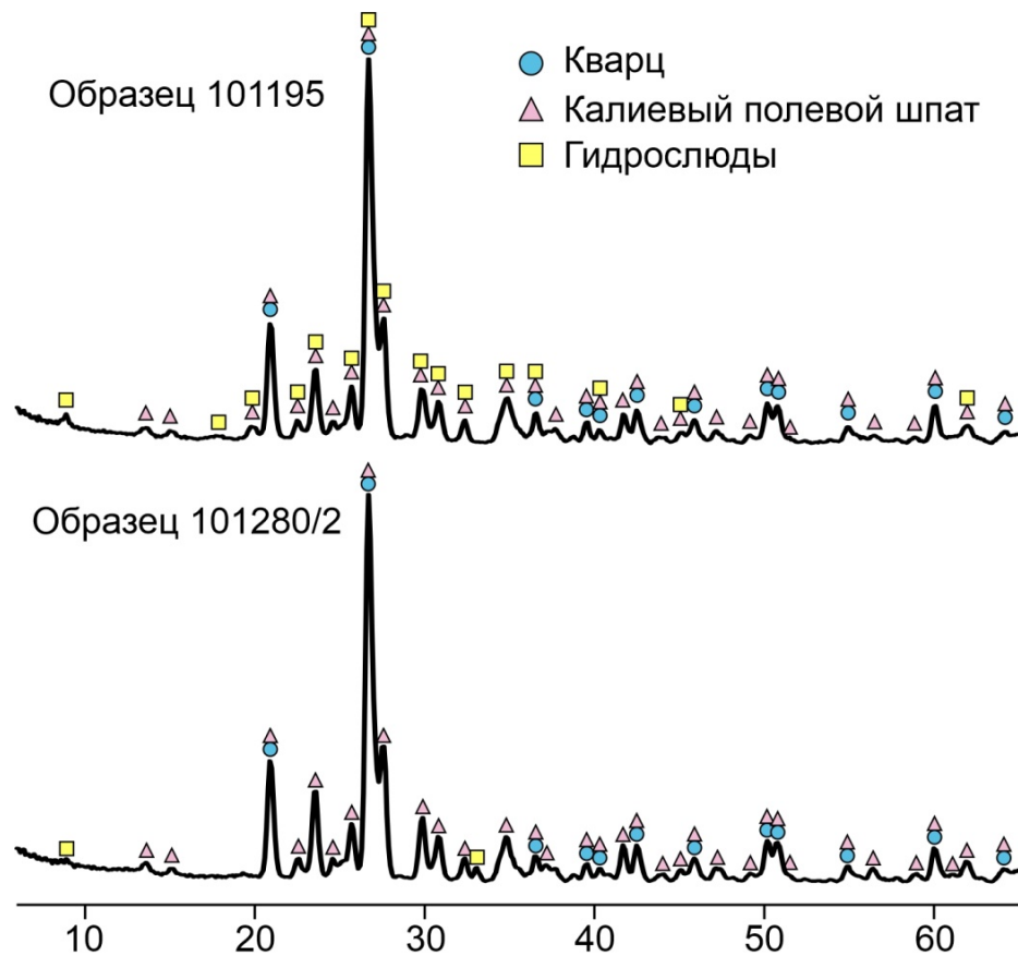
Рис. 2.9. Порошковые рентгеновские дифрактограммы представительных образцов калиевополевошпат-кварцевых метасоматитов, развивающихся по риодацитам толятовьямского комплекса.
