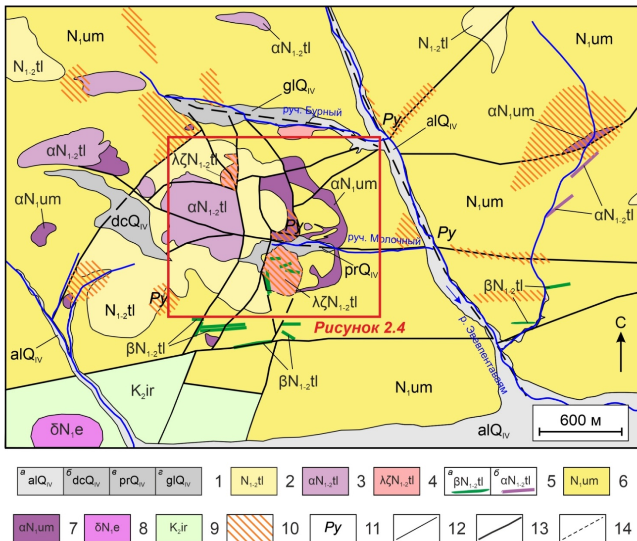
Рис. 2.3. Схема геологического строения рудопроявления Эвепента (составлена по материалам Л. А. Безруковой с соавторами (2004ф) с дополнениями и упрощениями). 1 – четвертичные отложения (а – аллювиальные, б – делювиальные, в – пролювиальные, г – гляциальные); 2 – покровные образования толятоваямского вулканического комплекса; 3 – субвулканические андезиты толятоваямского комплекса; 4 – субвулканические дациты и риодациты толятоваямского комплекса; 5 – дайки толятоваямского комплекса (а – базальтового состава, б – андезитового состава); 6 – покровные образования умуваямского вулканического комплекса; 7 – субвулканические тела андезитов умуваямского комплекса; 8 – шток диоритов эмиваямского плутонического комплекса; 9 – вулканогенно-осадочные образования ирунейского комплекса; 10 – зоны аргиллизации и окварцевания; 11 – зоны пиритизации; 12 – границы геологических подразделений; 13 – разломы, выходящие на дневную поверхность; 14 – разломы предполагаемые, скрытые под четвертичными отложениями.
