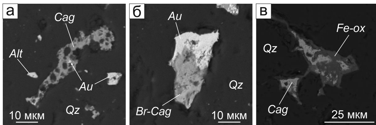
Рис. 4.15. Морфология зерен и взаимоотношения хлораргирита с другими минералами: а – хлораргирит в полости в кварце с реликтовым золотом; б – бромсодержащий хлораргирит, замещающий (?) самородное золото; в – срастание хлораргирита и гидроксидов железа в полости в кварце. Изображения в обратно-рассеянных электронах. Alt – алланит, Cag – хлораргирит, Au – самородное золото, Qz – кварц, Br-Cag – бромсодержащий хлораргирит, Fe-ox – гидроксиды железа.
