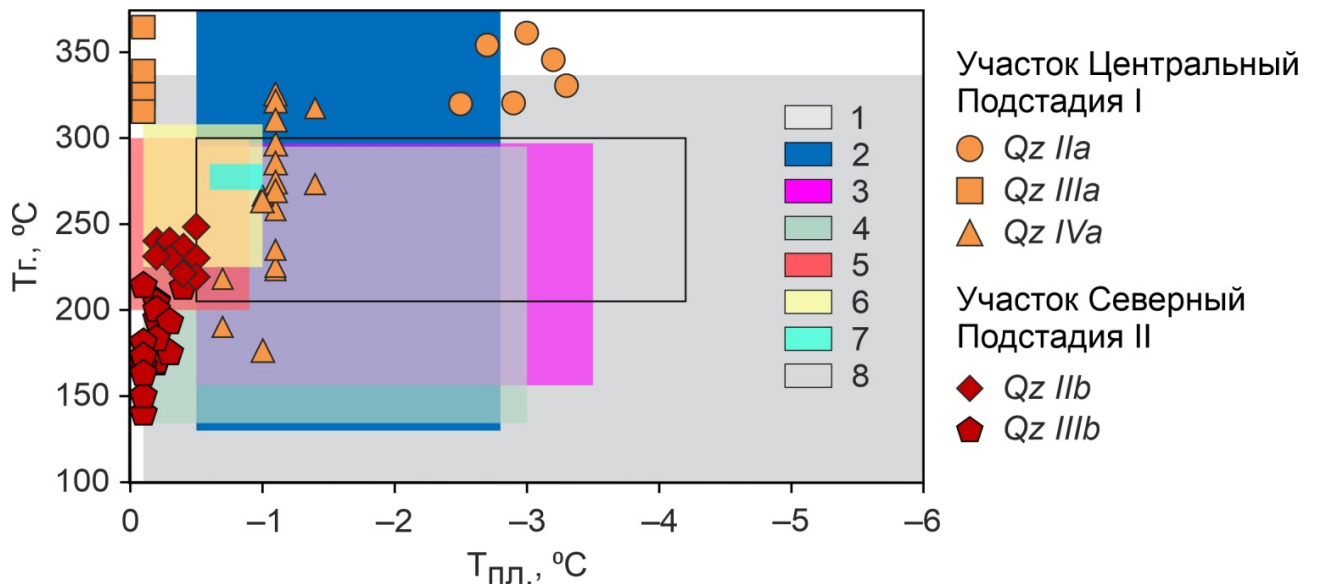
Рис. 5.6. Диаграмма зависимости температуры гомогенизации флюидных включений от температуры плавления льда для рудопроявления Эвепента и эпитегрмальных золото-серебряных объектов полуострова Камчатка: 1 – Асачинское (Takahashi et al., 2007; Боровиков и др., 2009); 2 – Родниковое (Takahashi et al., 2002; Tolstykh et al., 2022а); 3 – Мутновское (Takahashi et al., 2006); 4 – Малетойваям (Sidorov et al., 2020; Shapovalova et al., 2025); 5 – Агинское (Andreeva et al., 2013); 6 – Бараньевское (Tolstykh et al., 2021; Якич и др., 2022; Shapovalova et al., 2025); 7 – Лазурное (Shapovalova et al., 2025); 8 – Кумроч (Shapovalova et al., 2025).
