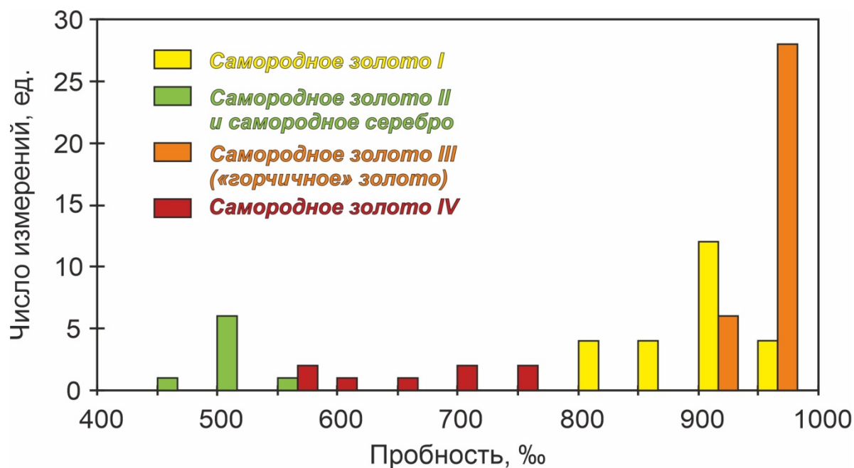
Рис. 4.11. Гистограмма распределения частот пробности самородного золота и серебра для участка Центральный рудопроувления Эвепента.
