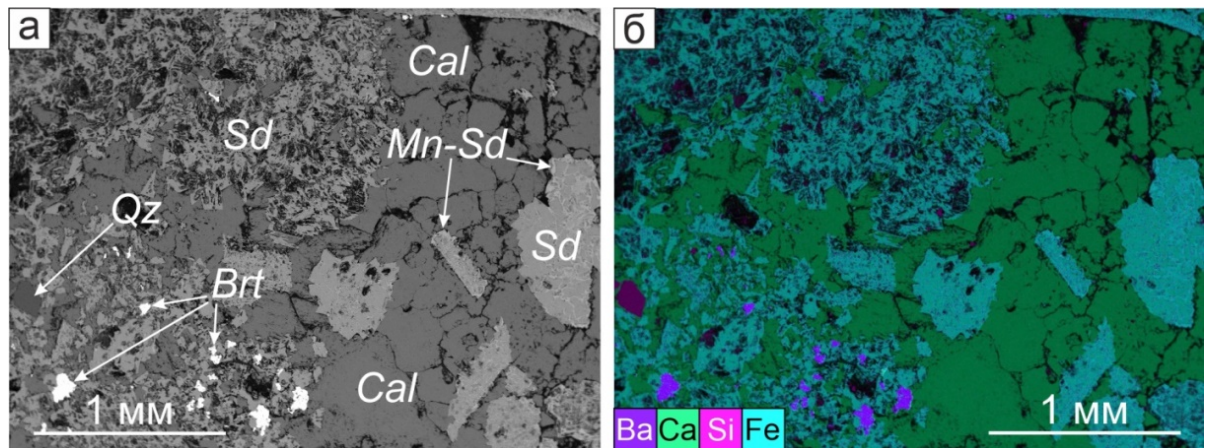
Рис. 4.27. Карбонатная минеральная ассоциация и минеральные взаимоотношения: а – изображение в обратно-рассеянных электронах; б – карта элементного состава. Cal – кальцит, Sd – сидерит, Mn-Sd – марганецсодержащий сидерит, Qz – кварц, Brt – барит.
