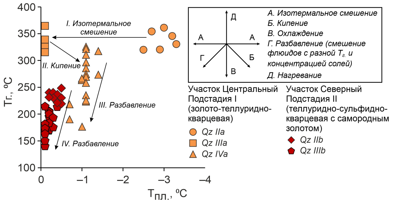
Рис. 5.5. Диаграмма зависимости температуры гомогенизации от температуры плавления льда. На врезке пути эволюции флюида, обусловленные различными геологическими процессами, показаны по данным (Wilkinson, 2001).
