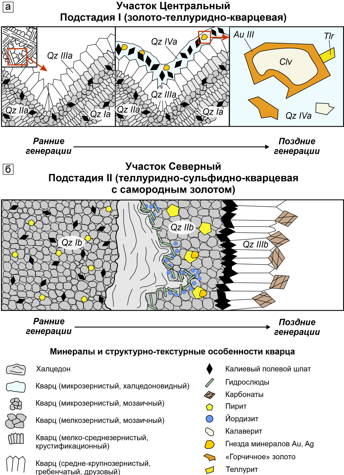
Рис. 4.34. Схема минеральных взаимоотношений и структурно-текстурных особенностей рудных калиевополевошпат-кварцевых жил: а – подстадия I; б – подстадия II. Qz Ia , Qz IIa , Qz IIIa , Qz IVa – кварц первой, второй, третьей и четвертой генерации, соответственно, в жилах ранней подстадии, Au III – самородное золото третьей разновидности («горчичное» золото), Clv – калаверит, Tlr – теллурит, Qz Ib , Qz IIb , Qz IIIb – кварц первой, второй и третьей генерации, соответственно, в жилах поздней подстадии.
