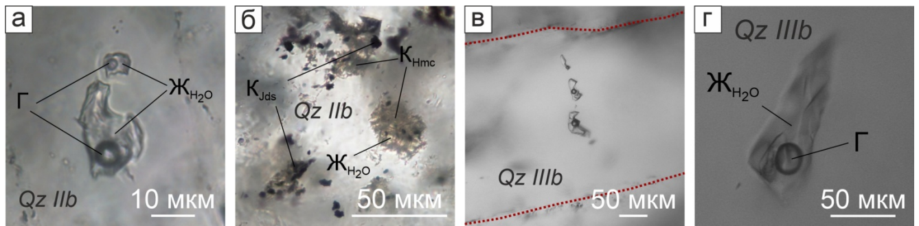
Рис. 5.2. Типы первичных флюидных включений в кварце IIb (а, б) и IIIb (в, г) из рудных жил подстадии II (теллуридно-сульфидно-кварцевой с самородным золотом): а – ассоциация двухфазных газовой-жидких включений; б – двухфазные кристалло-флюидные включения; в – ассоциация двухфазных газовой-жидких включений (красными линиями показаны границы кристалла кварца); г – двухфазное газовой-жидкое включение. Qz – кварц, \text{Ж}_{\text{H}_2\text{O}} – жидкая фаза (вода), Г – газовая фаза, \text{K}_{\text{Hmc}} – кристаллическая фаза (минералы группы гидрослюд), \text{K}_{\text{Jds}} – кристаллическая фаза (йордизит).
