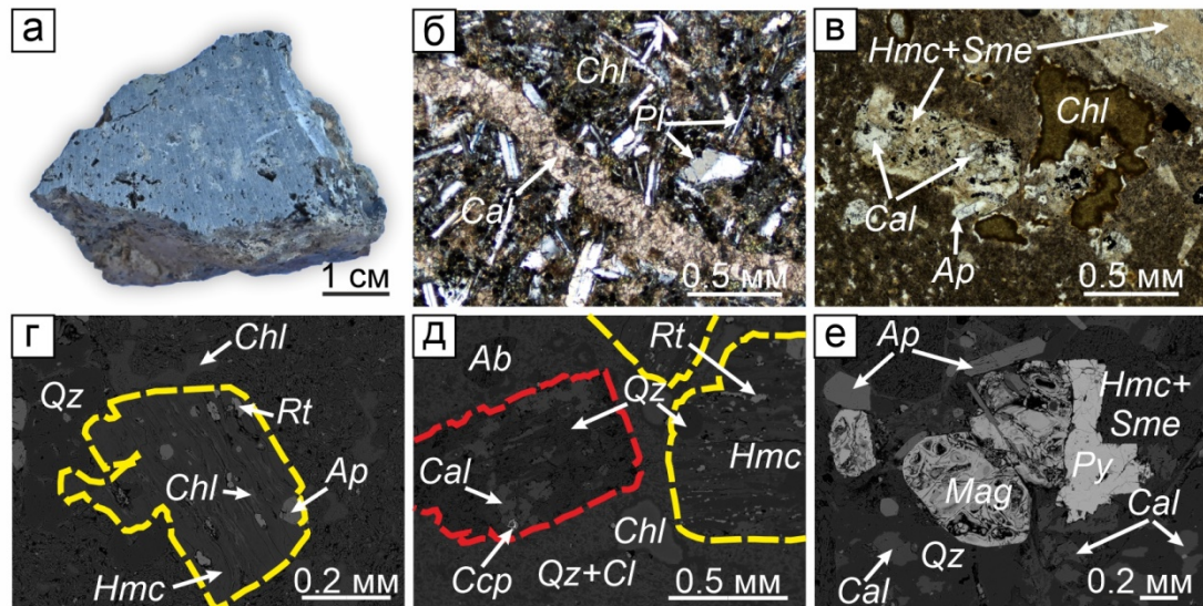
Рис. 2.6. Пропилиты по андезитам: а – фото образца; б – карбонатный прожилок в пропилитизированном базальте (дайка); в – глинистые минералы, кальцит и апатит по плагиоклазу; г – глинистые минералы, хлорит, апатит и рутил по биотиту (желтые контуры); д – кальцит и кварц по плагиоклазу (красный контур), кварц, глинистые минералы и рутил по биотиту (желтые контуры); е – пирит, обрастающий реликтовый магнетит. Изображение (б) в проходящем свете с анализатором, (в) – в проходящем свете без анализатора; (г–е) – изображения в обратно-рассеянных электронах. Chl – хлорит, Pl – плагиоклаз, Cal – кальцит, Hmc – минералы группы гидрослюдов, Sme – минералы группы смектитов, Ap – апатит, Qz – кварц, Rt – рутил, Ab – альбит, Ccp – халькопирит, Mag – магнетит, Pu – пирит.
