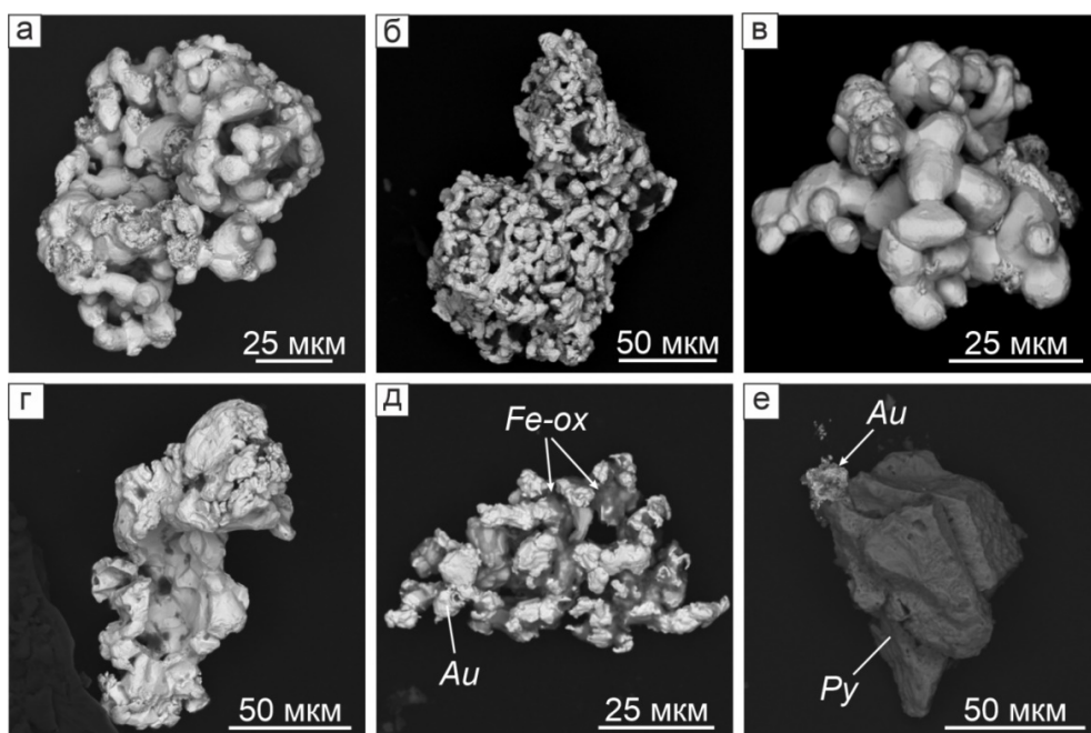
Рис. 4.9. Морфологические особенности сростков самородного золота I и II: а–в – зерна дендритовидной формы; г – дендритовидное зерно с отпечатками граней жильных минералов; д – дендритовидное зерно с присыпкой гидроксидов железа; е – зерно золота в сростании с пиритом. Изображения во вторичных электронах. Au – самородное золото, Fe-ox – гидроксиды железа, Py – пирит.
