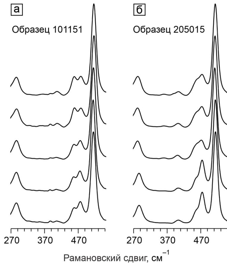
Рис. 4.31. Сравнение полос в области 270–550 \text{см}^{-1} в КР-спектрах различных зерен калиевого полевого шпата в пределах одной генерации: а – участок Центральный; б – участок Северный.
