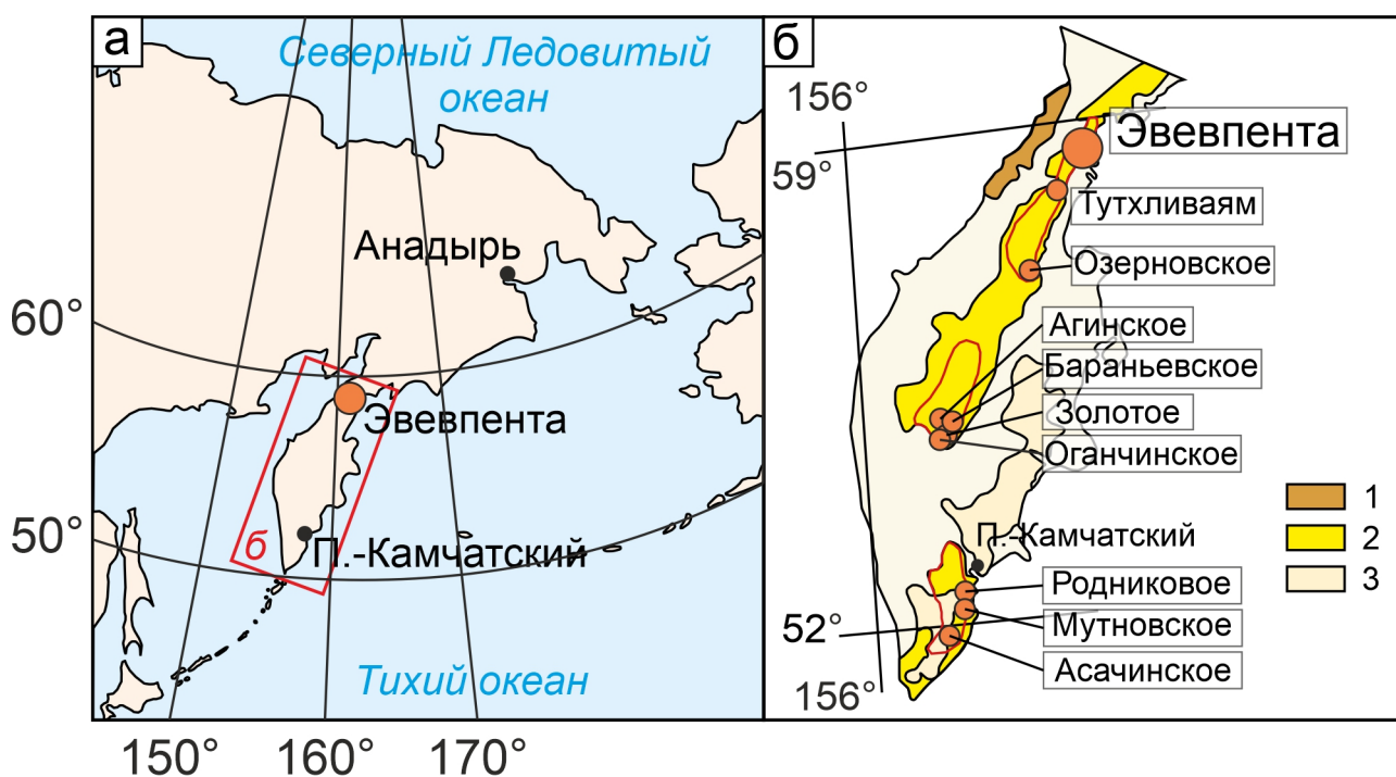
Рис. 1.1. Схема расположения эпитермального золото-серебряного рудопроявления Эвевпента: а – географическое положение полуострова Камчатка; б – местоположение рудопроявления Эвевпента на полуострове Камчатка. Вулканогенные пояса Камчатки по (Петренко, 1999): 1 – Западно-Камчатский, 2 – Центрально-Камчатский и 3 – Восточно-Камчатский. Красными контурами на (б) обозначены Северо-Камчатский, Центрально-Камчатский и Южно-Камчатский рудные районы.
