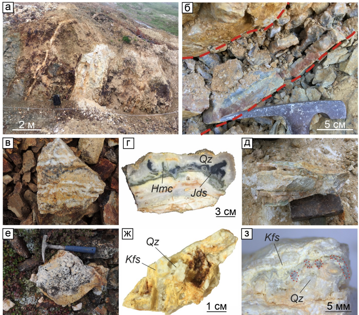
Рис. 4.1. Текстуры особенностей жил и прожилков: а – калиевополевошпат-кварцевая жила участка Центральный; б – кварцевый прожилок участка Северный (красные штрихи – границы прожилка); в, г – образцы жил колломорфно-полосчатой текстуры; д – кварцевые прожилки крустификационной текстуры; е, ж – образцы калиевополевошпат-кварцевых жил каркасно-пластинчатой текстуры; з – черные гнезда, насыщенные рудными минералами в образце калиевополевошпат-кварцевой жилы (красные штрихи – границы гнезд). Hmc – минералы группы гидрослюд, Qz – кварц, Jds – йордизит, Kfs – калиевый полевой шпат.
