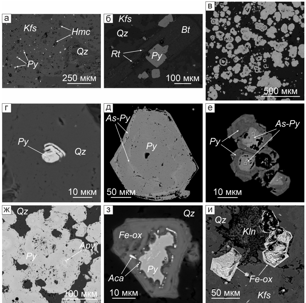
Рис. 4.2. Особенности морфологии и внутреннего строения пирита: а – рассеянная вкрапленность пирита в калиевополевошпат-кварцевом метасоматите; б – пирит в ассоциации с рутилом по порфировому вкрапленнику биотита в аргиллизированном риодаците; в – зерна пирита округлого фрамбоидального облика; г – скелетный кристалл пирита; д, е – зерна мышьяк содержащего пирита с осцилляционной зональностью; ж – включение арсенопирита в пирите; з – включения акантита в окисленном пирите; и – псевдоморфозы гидроксидов железа по пириту. Изображения в обратно-рассеянных электронах. Kfs – калиевый полевошпат, Hmc – минералы группы гидрослюд, Qz – кварц, Py – пирит, Bt – биотит, Rt – рутил, As-Py – мышьяк содержащий пирит, Apy – арсенопирит, Fe-ox – гидроксиды железа, Aca – акантит, Kln – минералы подгруппы каолинита.
