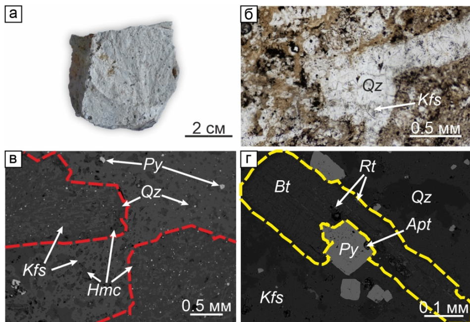
Рис. 2.10. Калиевополевошпат-кварцевые метасоматиты по риодацитам: а – фото образца; б – калиевополевошпат-кварцевый прожилок; в – агрегат глинистых минералов, кварца и пирита по плагиоклазу (красные контуры); г – реликтовый биотит, частично замещенный кварцем, рутилом, пиритом (желтые контуры). Изображение (б) в проходящем свете без анализатора; (в, г) – изображения в обратно-рассеянных электронах. Qz – кварц, Kfs – калиевый полевой шпат, Py – пирит, Hmc – минералы группы гидрослюды, Rt – рутил, Bt – биотит, Apt – апатит.
