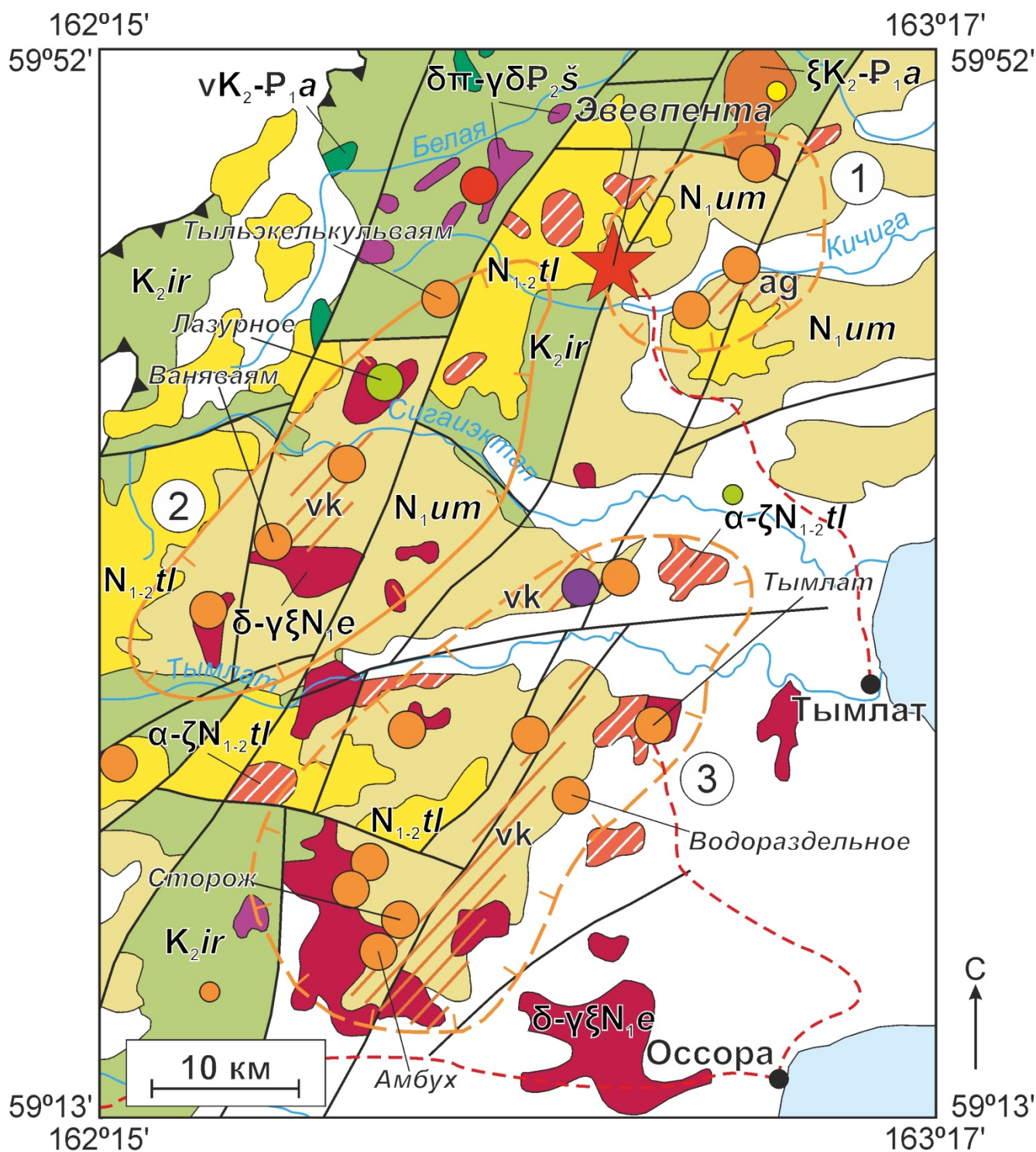
Рис. 2.1. Схематическая карта закономерностей размещения полезных ископаемых для северной части Северо-Камчатского рудного района. Составлена автором с использованием материалов (Карта..., 1999; Безрукова и др., 2004ф; Сляднев..., 2013).
