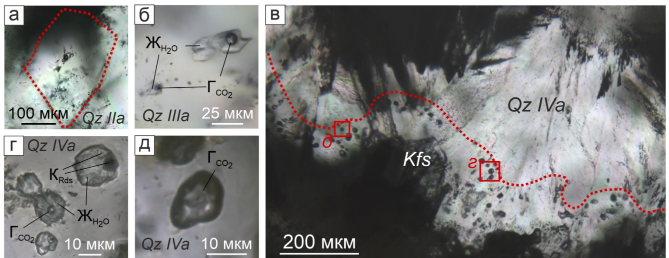
Рис. 5.1. Типы первичных флюидных включений в кварце IIa и IIIa (а, б), а также в кварце IVa (в–д) из рудных жил подстадии I (золото-теллуридно-кварцевой): а – флюидное включение в центральной части зерна кварца (красными линиями показана граница зерна); б – ассоциация флюидных включений, состоящая из двухфазных газовой-жидких включений; в – зонально расположенные флюидные включения в халцедоновидном кварце (красными линиями показана зона роста); г – ассоциация двухфазных газовой-жидких и многофазных кристалло-флюидных включений; д – однофазное газовое включение. Qz – кварц, Kfs – калиевый полевошпат, Ж H2O – жидкая фаза (вода), Г CO2 – газовая фаза (углекислый газ), K Rds – кристаллическая фаза (родохрозит).
