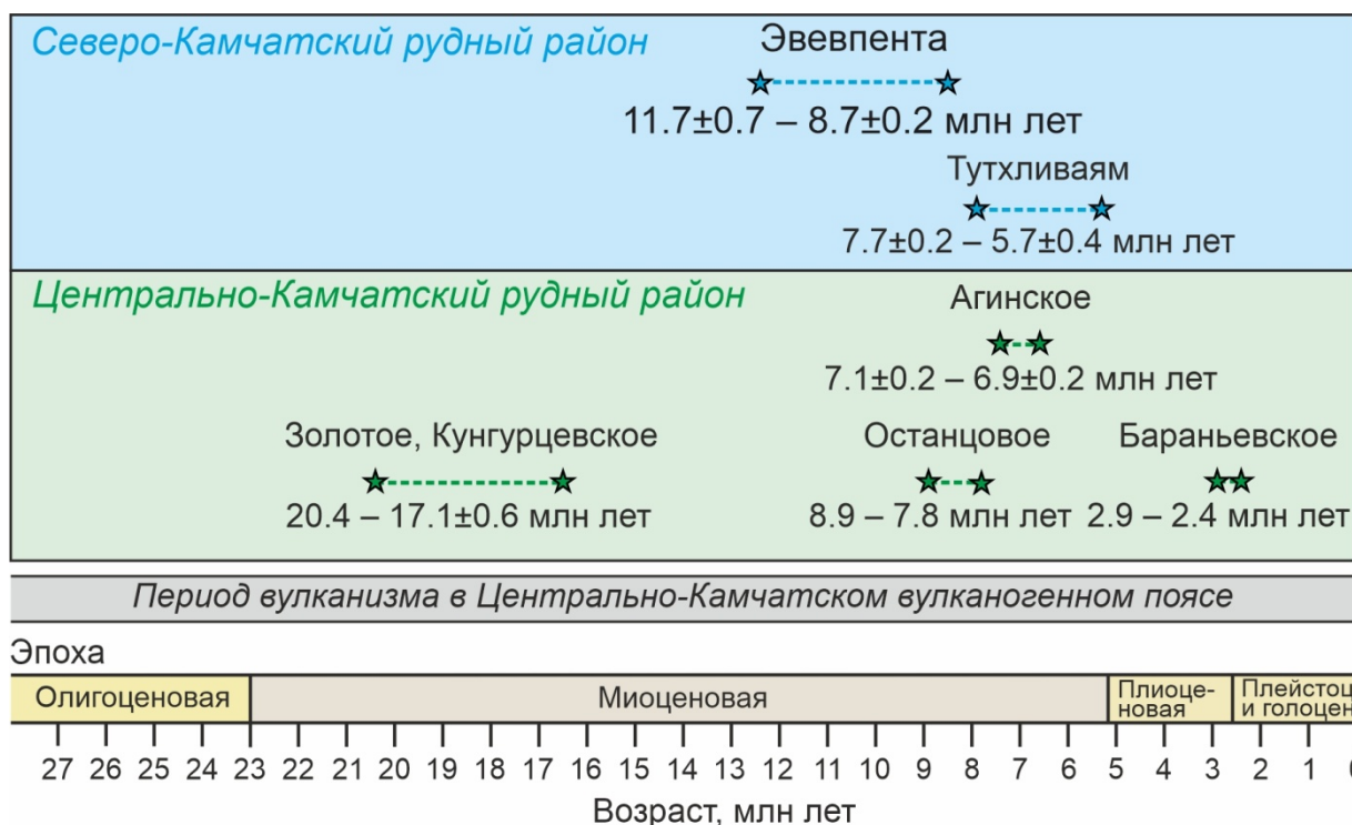
Рис. 3.6. Диаграмма возраста эпитермальных Au–Ag месторождений Центрально Камчатского вулканогенного пояса (К–Аг метод, по калиевому полевому шпату из рудных жил). Возраст рудопроявления Эвевпента указан по данным настоящего исследования, рудопроявления Тутхливаям – по (Швейгерт и др., 2026), месторождений Центрально-Камчатского рудного района по (Большаков и др., 2010; Округин, Шишканова, 2013; Andreeva et al., 2013; Takahashi et al., 2013).
