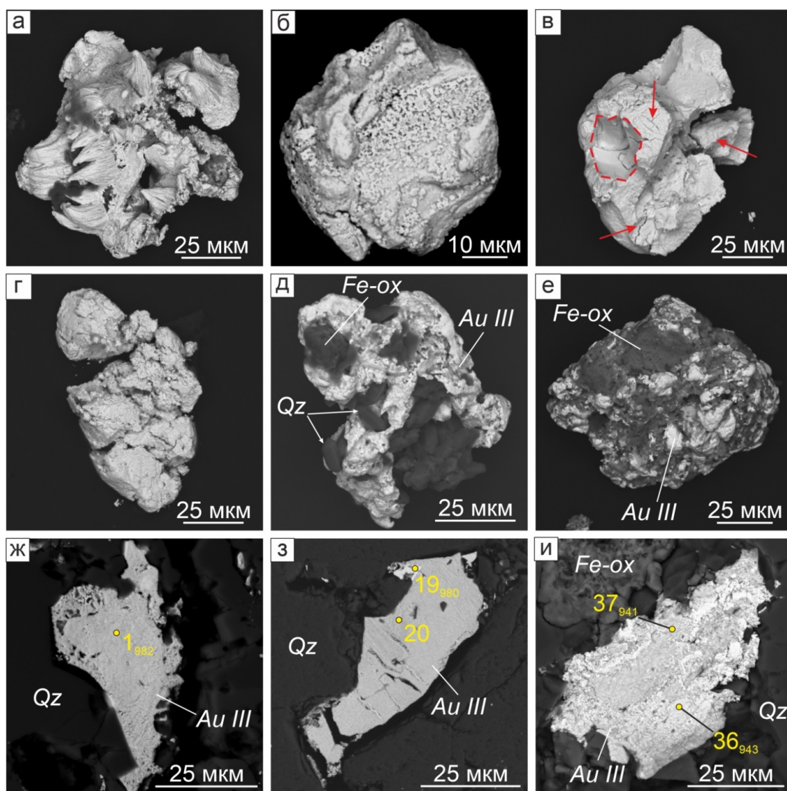
Рис. 4.13. Особенности морфологии и внутреннего строения «горчичного» самородного золота III: а, б – зерна «горчичного» золота с наростами самородного золота; в, г – хрупкие трещиноватые зерна, красный контур – след от иглы, стрелки указывают на трещины и обломок зерна, возникшие после механического воздействия; д, е – зерна, покрытые «рубашкой» из гидроксидов железа; ж – зерно пористого внутреннего строения; з – зерно колломорфной текстуры в сростании с сульфидами Au–Ag и участками высокопробного золота однородного внутреннего строения (белое); и – зерно с участками, насыщенными гидроксидами железа (светло-серое). На изображениях ж–и желтые круги – аналитические точки, номера соответствуют номерам анализов в табл. 4.7 , индексы – пробность. Изображения во вторичных электронах (а–е) и в обратно-рассеянных электронах (ж–и). Au III – самородное золото третьей разновидности («горчичное» золото), Qz – кварц, Fe-ox – гидроксиды железа.
