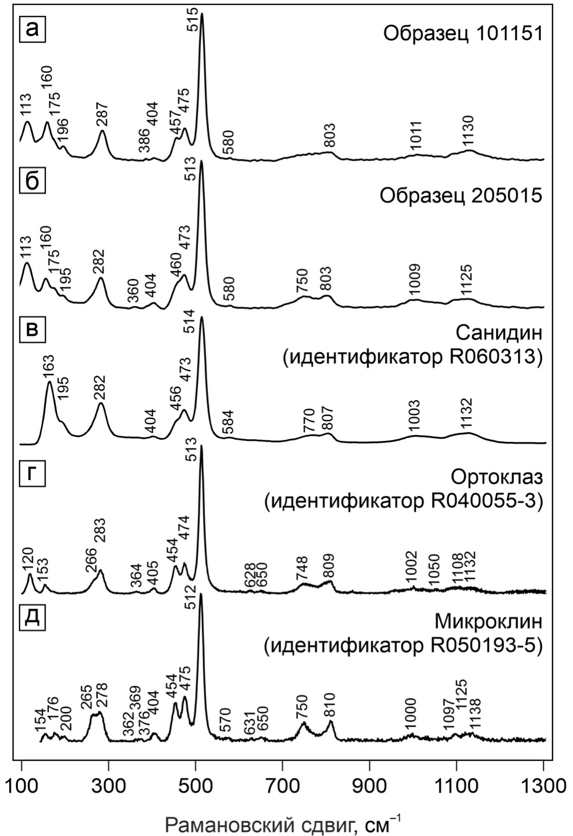
Рис. 4.30. КР-спектры калиевого полевого шпата: а, б – рудопроявление Эвепента, участки Центральный (а) и Северный (б); в–д – спектры санидина, ортоклаза и микроклина, соответственно, из базы данных RRUFF ( http://rruff.info ).
