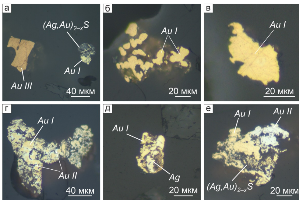
Рис. 4.8. Разновидности самородного золота: а – зерно самородного золота I в сростании с сульфидами Au–Ag и зерно самородного золота III («горчичное» золото); б – срез зерна самородного золота I дендритовидной формы; в – срез зерна самородного золота I комковидной формы; г – агрегат дендритовидной формы, в котором отдельные округлые кристаллы самородного золота I обрастают самородным золотом II; д – сростание золота I и самородного серебра; е – сростание самородного золота I с самородным золотом II и сульфидами Au–Ag. Фото в отраженном свете. Au I , Au II , Au III – самородное золото первой, второй и третьей разновидности соответственно.
