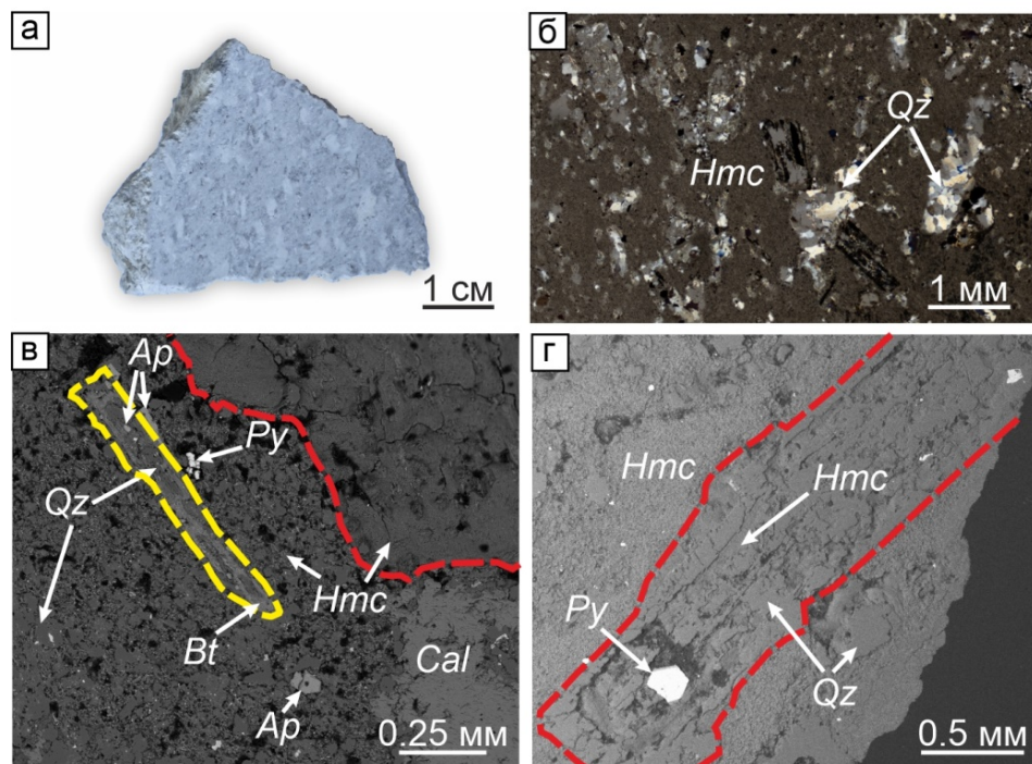
Рис. 2.8. Аргиллизиты по риодацитам: а – фото образца; б – реликтовая бластопорфировая структура породы; в – кварц по биотиту (желтый пунктир) и глинистые минералы по плагиоклазу (красный пунктир); г – кварц, глинистые минералы и пирит по плагиоклазу (красные контуры). Изображение (б) – в проходящем свете с анализатором; (в, г) – изображения в обратно-рассеянных электронах. Hmc – минералы группы гидрослюд, Qz – кварц, Ap – апатит, Bt – биотит, Cal – кальцит, Py – пирит.
