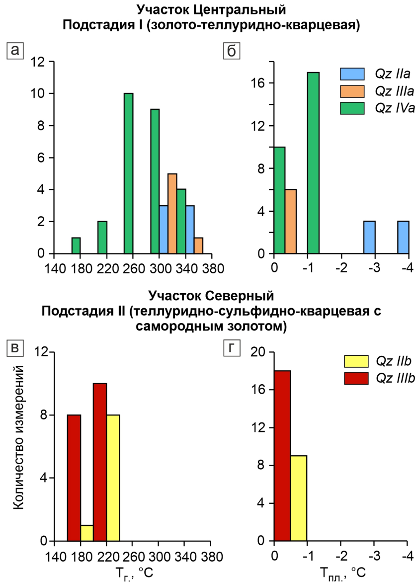
Рис. 5.4. Гистограммы распределения частот температур гомогенизации и плавления льда для первичных флюидных включений в кварце из рудных калиевополевошпат-кварцевых жил.
