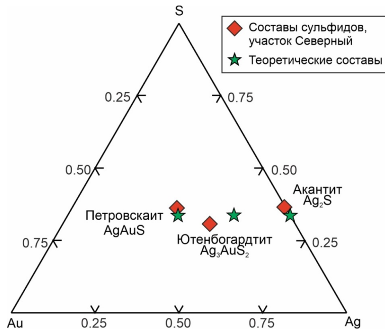
Рис. 4.22. Диаграмма химических составов (ат. %) минералов системы Au–Ag–S, участок Северный, рудопроявление Эвевпента.
