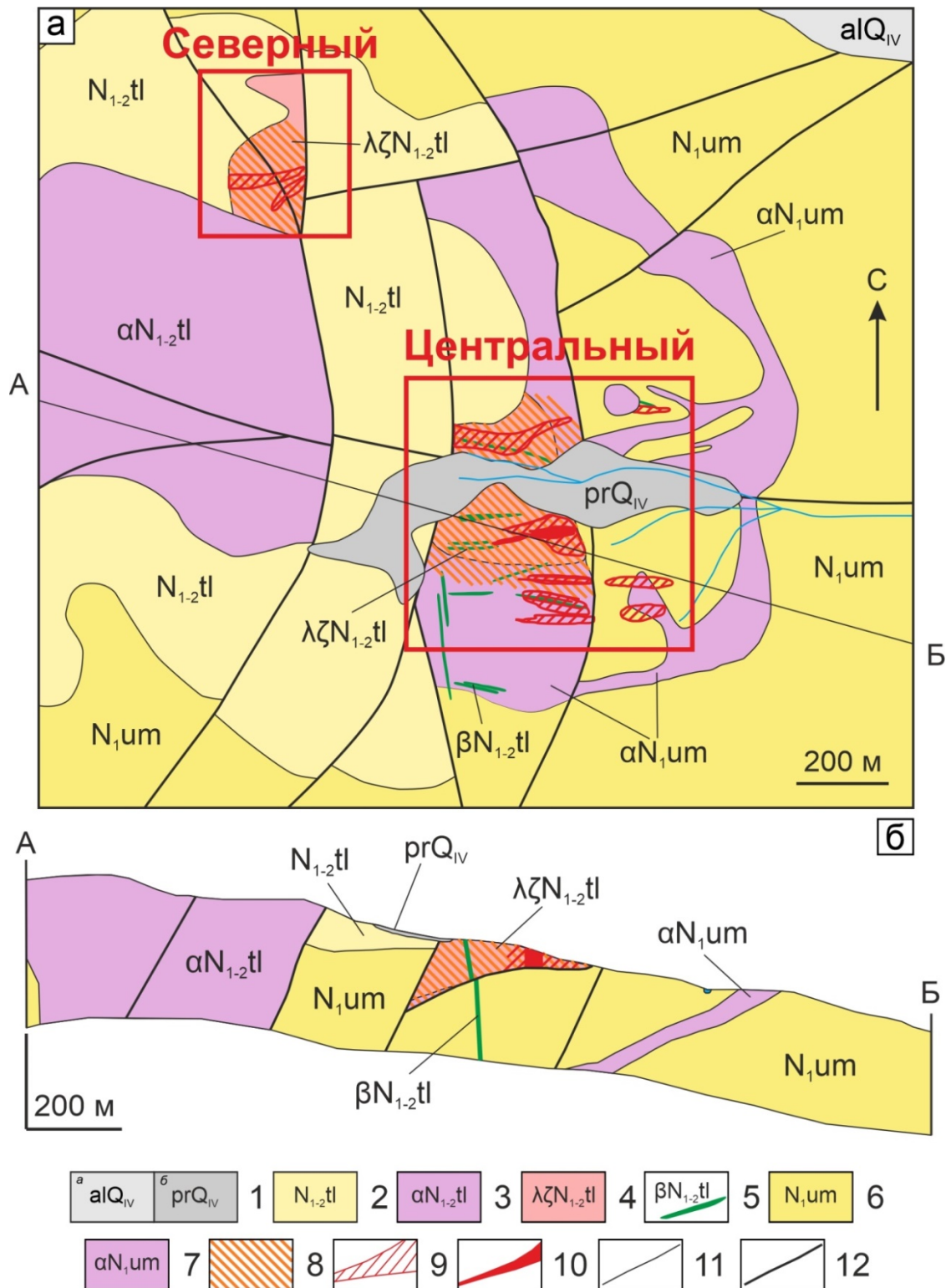
Рис. 2.4. Схема геологического строения участков Центральный и Северный рудопроявления Эвепента и разрез по линии АБ (Безрукова и др., 2004ф; Семериков и др., 2021ф с дополнениями и упрощениями). 1 – четвертичные отложения (а – аллювиальные, б – пролювиальные); 2 – покровные образования толятоваямского вулканического комплекса; 3 – субвулканические андезиты толятоваямского комплекса; 4 – субвулканические дациты и риодациты толятоваямского комплекса; 5 – дайки базальтов толятоваямского комплекса; 6 – покровные образования умуваямского вулканического комплекса; 7 – субвулканические тела андезитов умуваямского комплекса; 8 – зоны аргиллизации и окварцевания; 9 – зоны кварцевого прожилкования; 10 – кварцевые жилы; 11 – границы геологических подразделений; 12 – разломы, выходящие на дневную поверхность.
