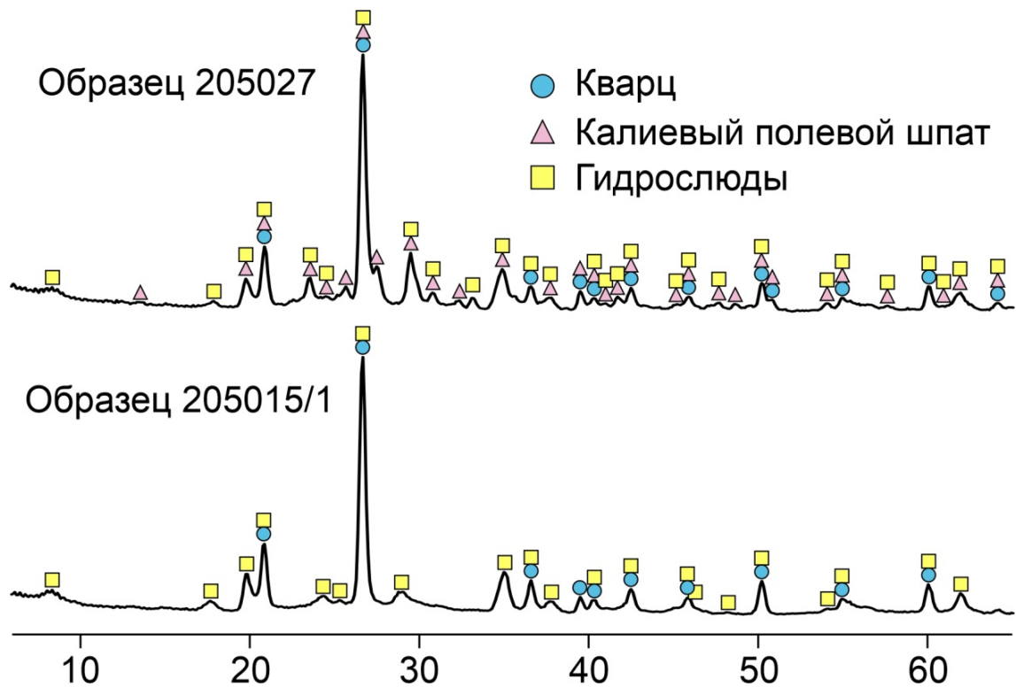
Рис. 2.7. Порошковые рентгеновские дифрактограммы представительных образцов аргиллизитов, развивающихся по риодацитам толятовьямского комплекса.
