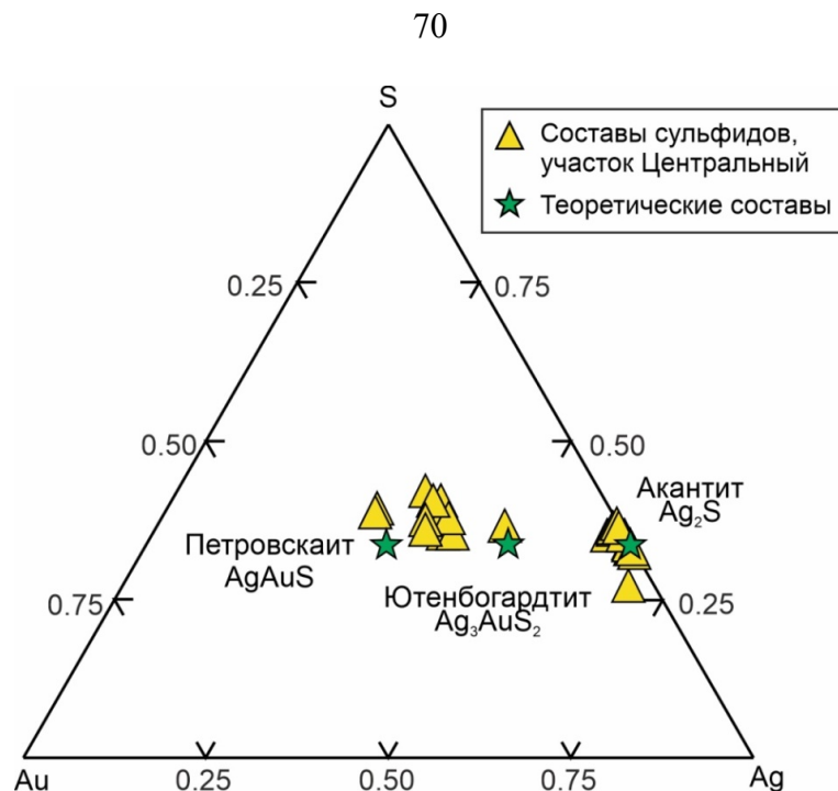
Рис. 4.5. Диаграмма химических составов (ат. %) минералов системы Au–Ag–S, участок Центральный, рудопоявление Эвепента.
