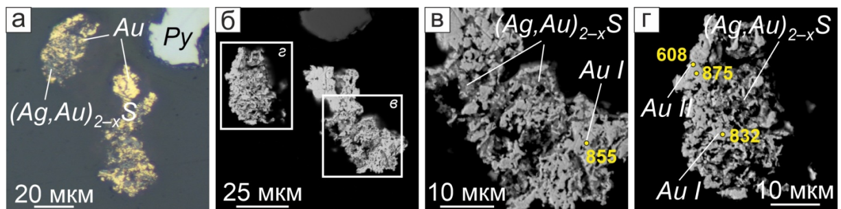
Рис. 4.25. Внутреннее строение дендритовидных агрегатов самородного золота I и II: а, б – агрегаты самородного золота I и II дендритовидной формы в ассоциации с фазами (\text{Ag,Au})_{2-x}\text{S} (в–г – участки детализации). Фото в отраженном свете (а) и изображения в обратно-рассеянных электронах (б–г). На рисунках (в, г) желтые круги – аналитические точки, числа – пробность самородного золота. Au – самородное золото, Py – пирит, Au I – самородное золото первой разновидности, Au II – самородное золото второй разновидности.
