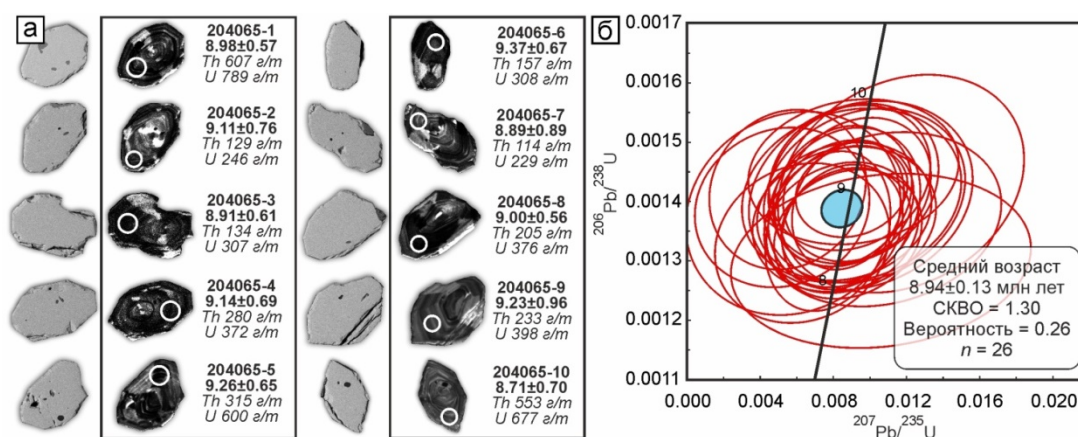
Рис. 3.2. Результаты U–Pb изотопного датирования первой группы кристаллов циркона, проанализированных методом ЛА-ИСП-МС: а – зональность и возраст цирконов; левый столбец – изображения в обратно-рассеянных электронах, правый столбец – катодолуминесцентные изображения, белые круги – область анализа; б – диаграмма с конкордией, красные эллипсы – единичные измерения для разных кристаллов циркона и их зон с погрешностью 2σ, синий эллипс – средневзвешенное значение возраста конкордии с погрешностью 2σ.
