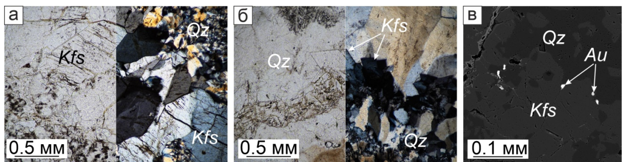
Рис. 4.16. Калиевый полевой шпат из золотоносных калиевополевошпат-кварцевых жил и прожилков: а – кристаллы калиевого полевого шпата с прямоугольными сечениями; б – кристаллы калиевого полевого шпата с ромбическими сечениями; в – ассоциация самородного золота в зоне прожилка, обогащенного калиевым полевым шпатом. Фотографии в проходящем свете (слева – без анализатора, справа – с анализатором) для (а, б) и изображение в обратно-рассеянных электронах для (в). Kfs – калиевый полевой шпат, Qz – кварц, Au – самородное золото.
