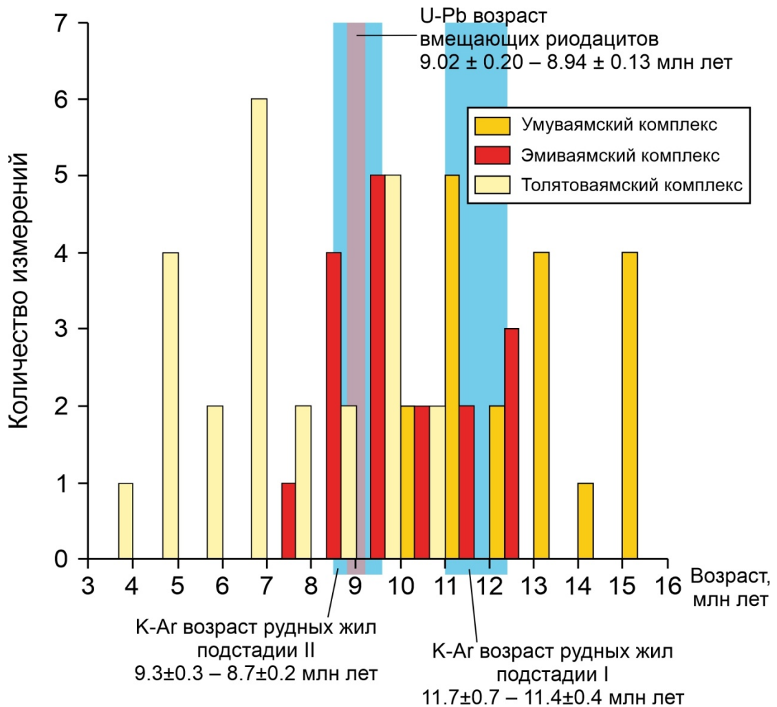
Рис. 3.5. Гистограмма распределения результатов датирования горных пород умуваямского и толятоваямского вулканических комплексов, а также эмиваямского плутонического комплекса Центрально-Камчатского вулканогенного пояса по данным (Боровцов и др., 1999ф; Федоров и др., 2025). Для сравнения показаны результаты изотопно-геохронологических исследований, полученные в данном исследовании.
