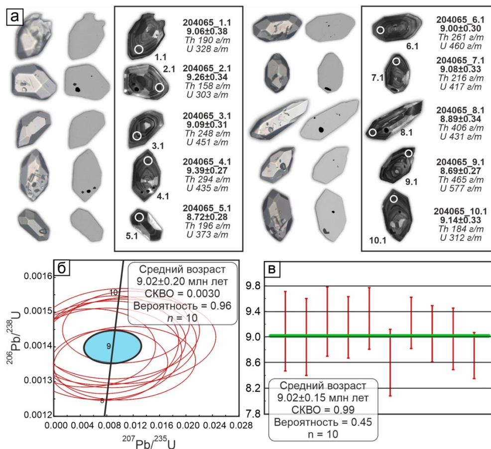
Рис. 3.3. Результаты U–Pb изотопного датирования второй группы кристаллов циркона, проанализированных на вторично-ионном микрозонде SHRIMP-II: а – морфология, зональность и возраст цирконов, левый столбец – фото в проходящем свете, центральный – изображения в обратно-рассеянных электронах, правый столбец – катодолуминесцентные изображения, белые круги – область анализа; б – диаграмма с конкордией, красные эллипсы – единичные измерения для разных кристаллов циркона и их зон с погрешностью 1σ, синий эллипс – средневзвешенное значение возраста конкордии с погрешностью 2σ; в – датировки с погрешностью 2σ индивидуальных кристаллов и средневзвешенное значение ^{206}\text{Pb}/^{238}\text{U} возраста.
