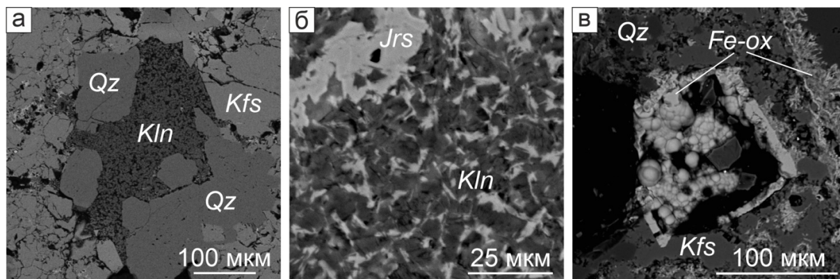
Рис. 4.18. Вторичные минералы зоны окисления: а – каолинит в полости в калиевополевошпат-кварцевой матрице; б – срастание ярозита и каолинита; в – почковидные, натечные агрегаты гидроксидов железа. Изображения в обратно-рассеянных электронах. Qz – кварц, Kln – минералы подгруппы каолинита, Kfs – калиевый полевой шпат, Jrs – ярозит, Fe-ox – гидроксиды железа.
