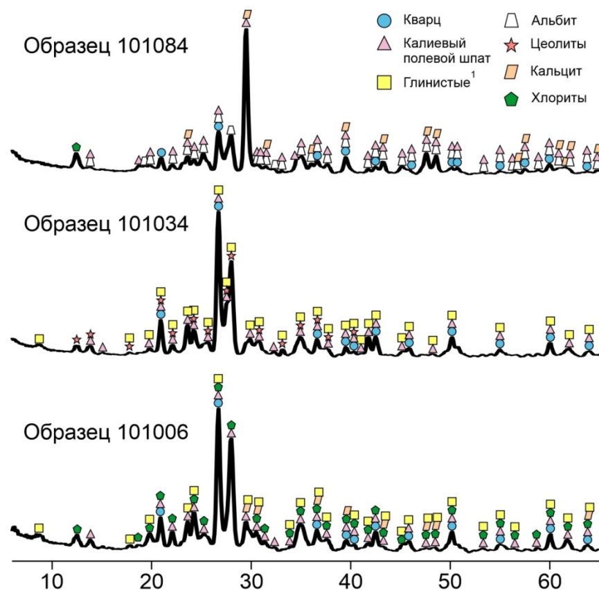
Рис. 2.5. Порошковые рентгеновские дифрактограммы представительных образцов пропилитов, развивающихся по андезитах умуваямского комплекса. 1 Минералы группы гидрослюд и смектитов.
