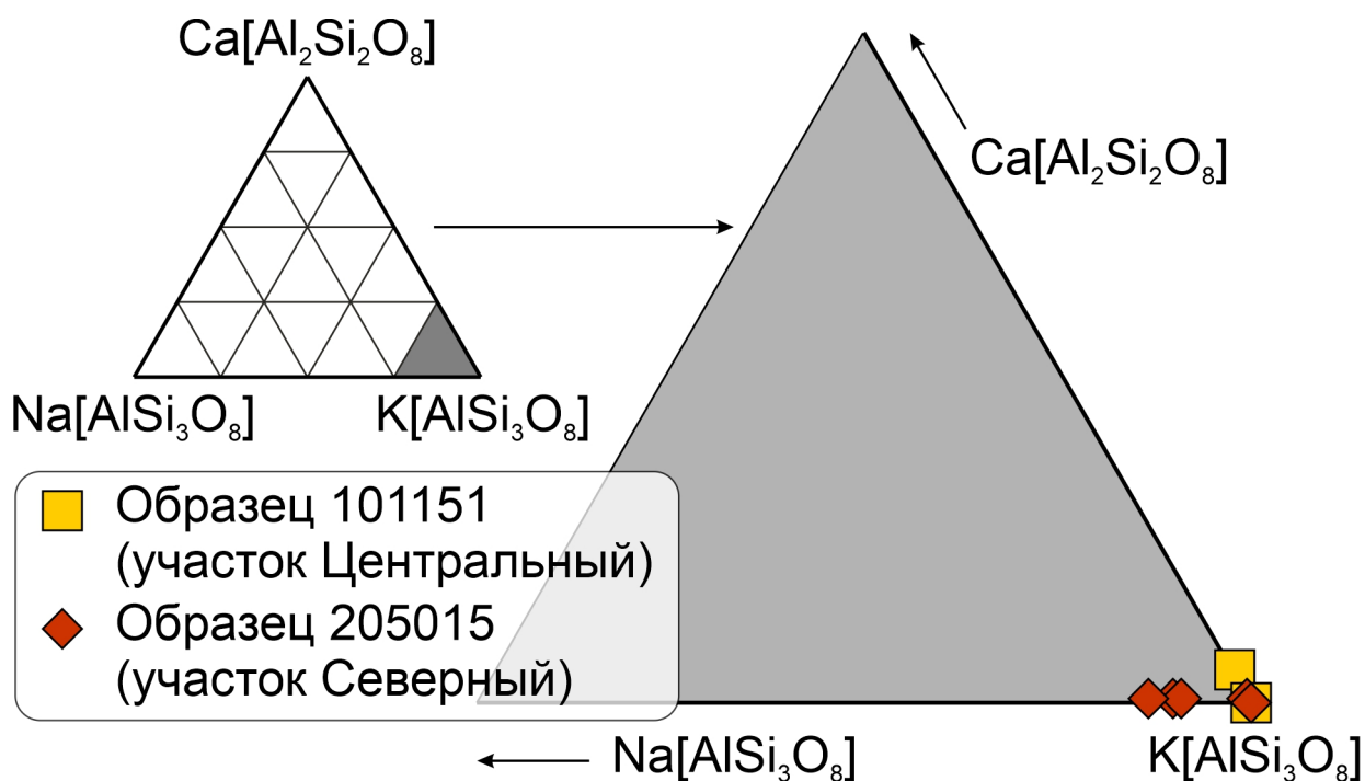
Рис. 4.29. Тройная диаграмма химического состава единичных анализов исследованных зерен калиевого полевого шпата рудопроявления Эвепента.
