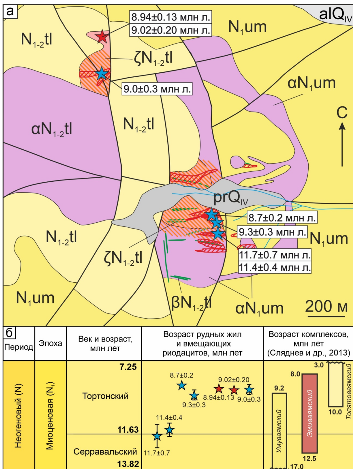
Рис. 3.4. Геологическая схема эпитермального рудопроявления Эввепента (а) и сопоставление изотопных возрастов (б). Схема (а) составлена по данным Л. А. Безруковой с соавторами (2004ф) и Л. А. Семерикова с соавторами (2021ф). На схеме (а) синими звездами отмечены места отбора проб из калиевополевошпат-кварцевых рудных жил с результатами К–Аг датирования; красной звездой – место отбора пробы вмещающих риодацитов с результатами U–Рb датирования. На изображении (б) показано сопоставление полученных возрастов. Остальные условные обозначения см. на рис. 2.4.
