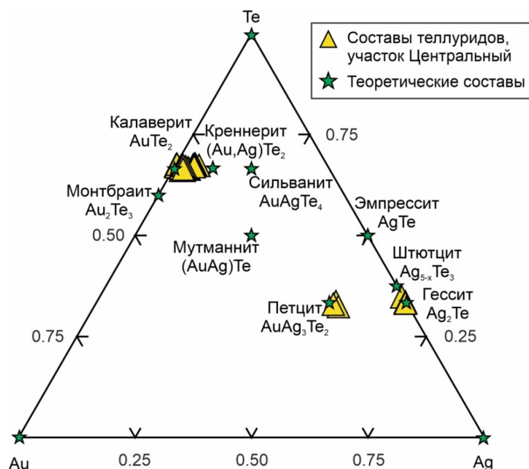
Рис. 4.7. Диаграмма составов (ат. %) минералов системы Au–Ag–Te, участок Центральный, рудопроявление Эвепента.
