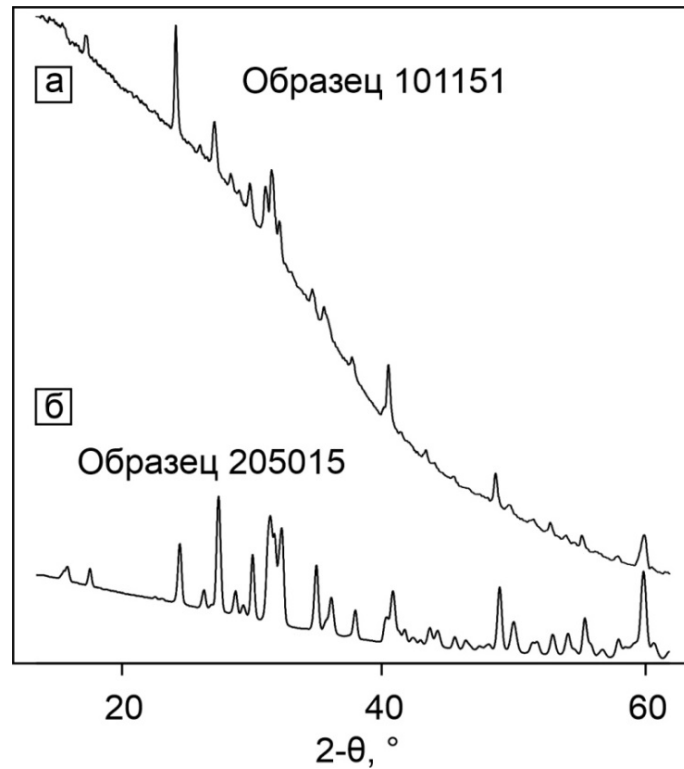
Рис. 4.32. Порошковые рентгенограммы калиевого полевого шпата: а – участок Центральный; б – участок Северный.
