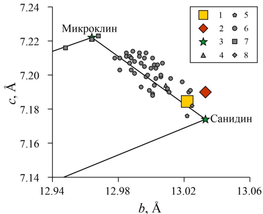
Рис. 4.33. Соотношение параметров b и c элементарной ячейки калиевого полевого шпата рудопроявления Эвепента и других эпитегрмальных месторождений адуляр-серицитового типа. 1 – рудопроявление Эвепента, участок Центральный, образец 101151 (наши данные), 2 – рудопроявление Эвепента, участок Северный, образец 205015 (наши данные), 3 – эталонные микроклин и санидин (Stewart, Wright, 1974), 4 – Хот Спрингс (США: Černý, Chapman, 1986), 5 – Гуанохуато (Мексика: Černý, Chapman, 1986), 6 – месторождения Квинсленда (Австралия: Dong, Morrison, 1995), 7 – Тапажос (Бразилия: Dreher et al., 1998), 8 – Хишикари (Япония: Zhou et al., 2001).
