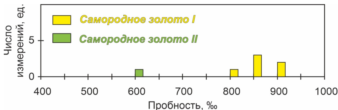
Рис. 4.26. Гистограмма распределения частот пробности самородного золота и серебра для участка Центральный рудопоявления Эвепента.
