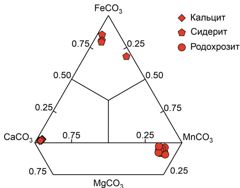
Рис. 4.28. Диаграмма \text{CaCO}_3\text{--MnCO}_3\text{--FeCO}_3\text{--MgCO}_3 составов карбонатов участка Северный, рудопроявление Эвевпента.
