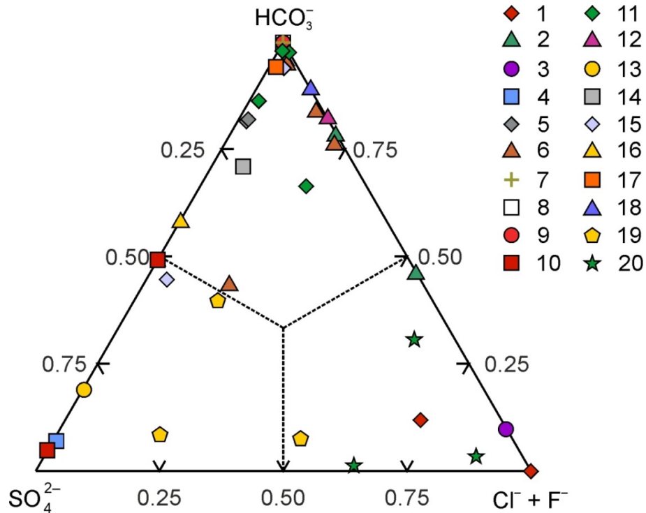
Рис. 5.7. Валовый анионный состав флюидных включений в кварце из эпитеермальных золото-серебряных месторождений адуляр-серицитового ( low-sulfidation ) типа на Северо-Востоке России, определенный методами газовой и ионной хроматографии в сочетании с ИСП-МС. 1 – Телевеем (Прокофьев и др., 2019; Бортников и др., 2022); 2 – Капелька (Прокофьев и др., 2019; Бортников и др., 2022); 3 – Джульетта (Колова и др., 2015; Прокофьев и др., 2015); 4 – Юное (Прокофьев и др., 2012б); 5 – Купол (Волков и др., 2012); 6 – Тихое (Колова и др., 2015; Волков и др., 2016а); 7 – Валунистое (Волков и др., 2020а); 8 – Огненный (Волков и др., 2019); 9 – Горный (Волков и др., 2019); 10 – Жильное (Волков и др., 2019); 11 – Двойное (Волков и др., 2018); 12 – Ольча (Волков и др., 2016б); 13 – Магнитное (Волков и др., 2016б); 14 – Биркачан (Волков и др., 2016б); 15 – Бургали (Волков и др., 2016б); 16 – Северное Бургали (Волков и др., 2016б); 17 – Южное Бургали (Волков и др., 2016б); 18 – Промежуточное (Волков, Прокофьев, 2011); 19 – Арыкеваам (Волков и др., 2020б); 20 – Каэнмываам (Волков и др., 2020б).
